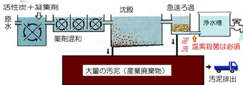
図10 急速ろ過のフロー
