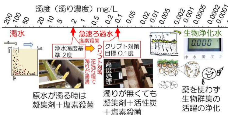
図28 水の濁りと処理水
