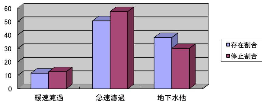
図2. 各浄水方法の占める割合と震災による停止割合 (複数の浄水システムが併存している浄水場を除外した場合)
